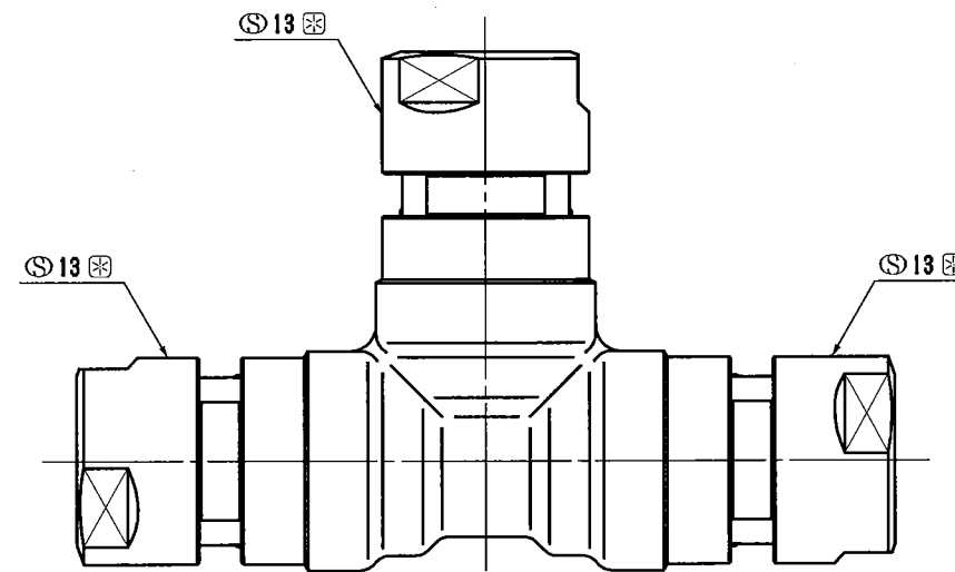
外觀図
