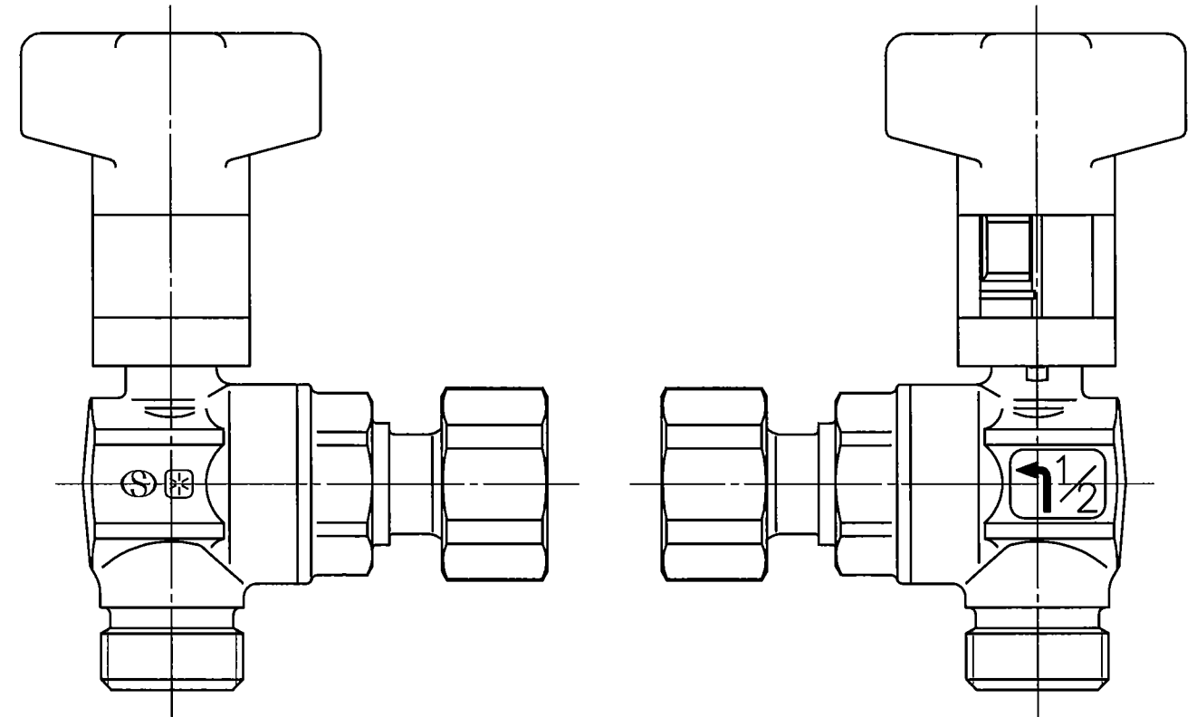
外觀図
